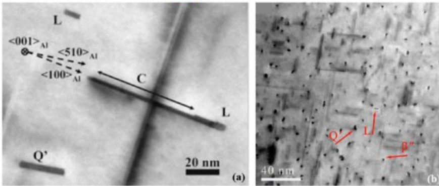
Microstructure d'un alliage Al-Mg-Si-Cu
