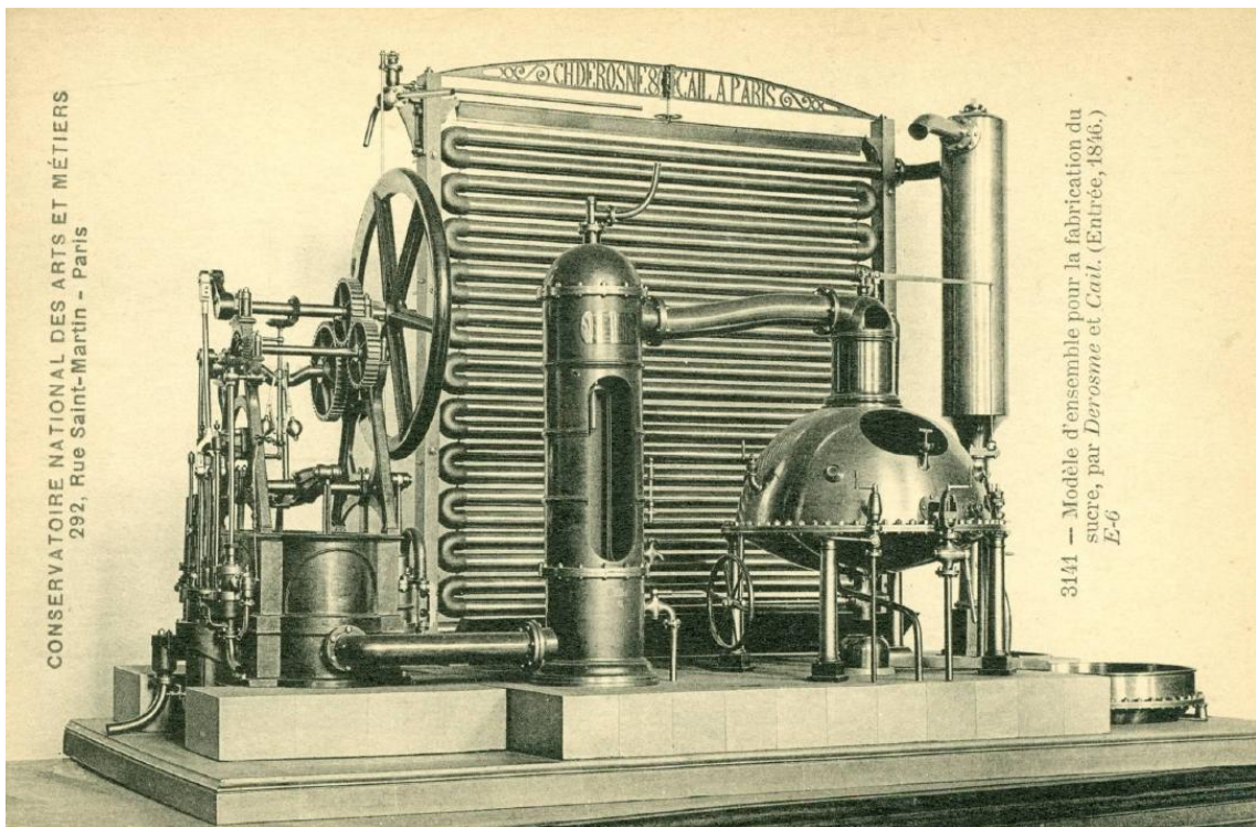
Modèles d'ensemble pour la fabrication du sucre par DEROSNE & CAIL Médaille d'or à l'Exposition Universelle de 1867
