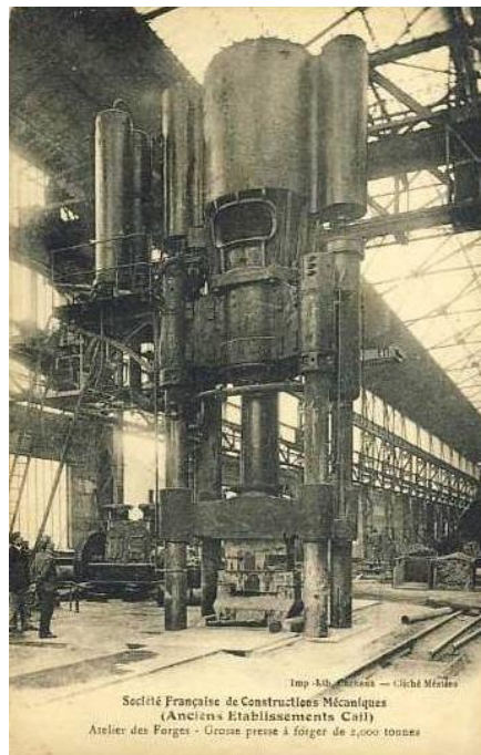
SFCM - Usines de Denain : Atelier des Forges - Grosse presse à fûter de 2,000 tonnes.
