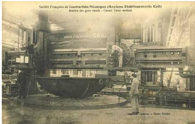
SFCM - Usines de Denain : Atelier des gros outils - Grand tour vertical.
